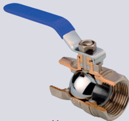
Vanne
