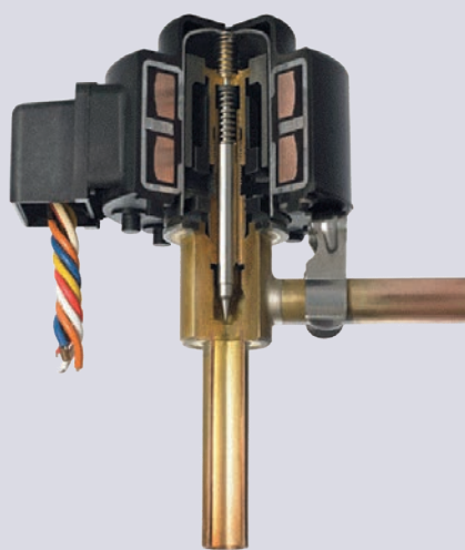
Détendeur
